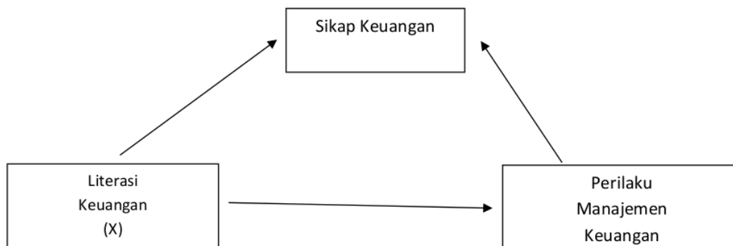
Gambar 1. Kerangka Penelitian
