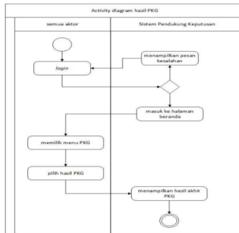
Gambar 3. Diagram Nol yang Diusulkan
