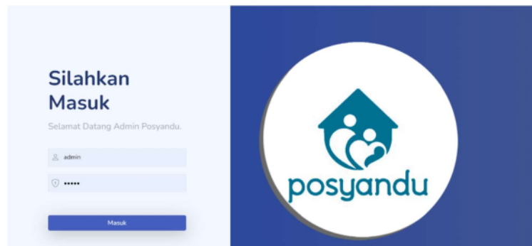
Gambar 3. 1 Halaman Login
