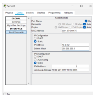
Gambar 6. Konfigurasi FastEthernet
