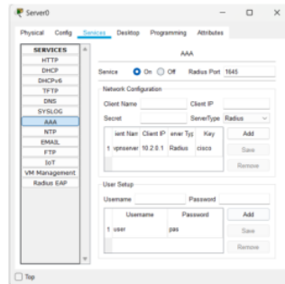
Gambar 6. Konfigurasi AAA
