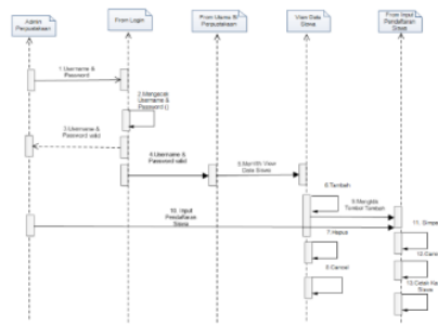
Gambar 8. Sequence Pendaftaran Siswa
