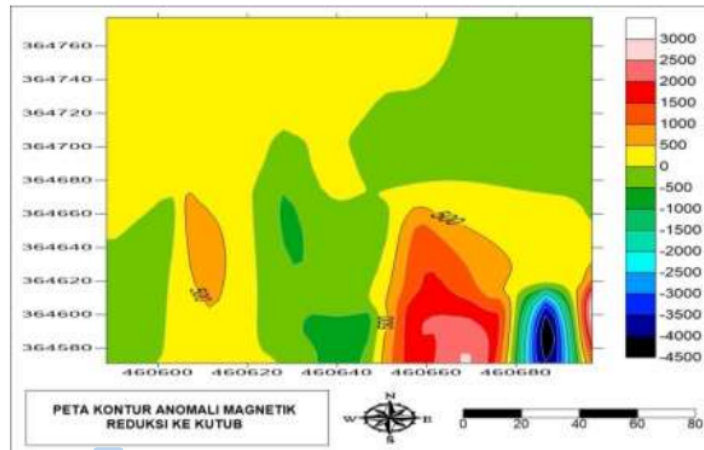
12 Gambar 3.3 Peta Kontur anomali reduksi ke kutub
