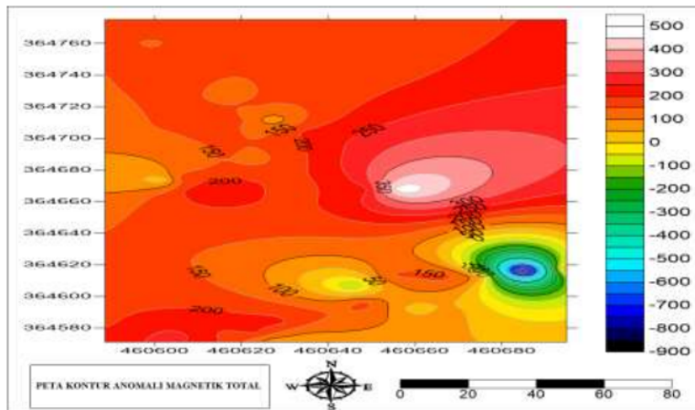
Gambar 3.2. Peta Kontur Anomali Medan Magnet Total.
