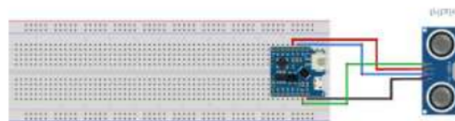
Gambar 5. Skematik Wemos D1 Mini Dengan Sensor Ultrasonik
