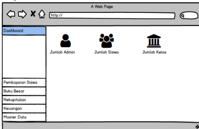
Gambar 8 1 Antarmuka Dashboard .
