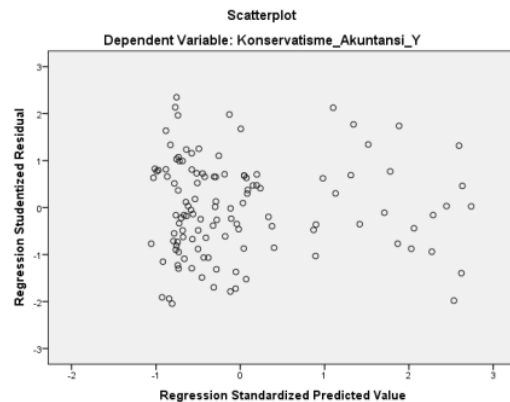
Gambar 3. Hasil Uji Heterokedastisitas Menggunakan Scatterplot
