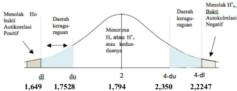
Gambar 4. Grafik Durbin-Watson
