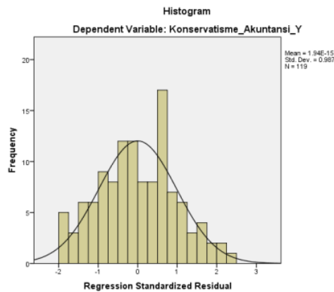
Gambar 2. Hasil Uji Normalitas Menggunakan Grafik Histogram
