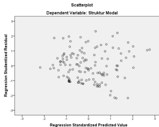
Gambar 3. Hasil Uji Heteroskedastisitas Menggunakan Grafik Scatterplot
