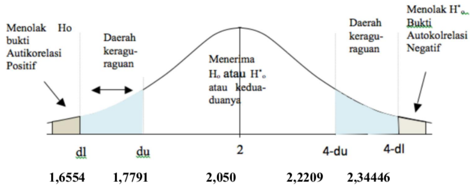
Gambar 4. Grafik Durbin-Watson
