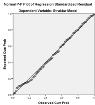
Gambar 1. Hasil Uji Normalitas Menggunakan Grafik Normal P-Plot
