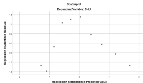
Gambar 1. Uji Heterokedastisitas
