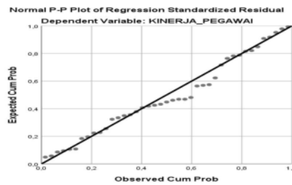
10 Gambar 1 Hasil Pengujian Uji Normalitas
