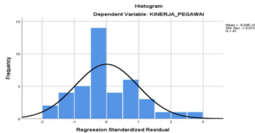
Gambar 2 Histogram Uji Asumsi Klasik
